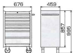
WS207R(S)(B)ローラーキャビネット寸法
