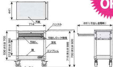
TC1701Rワークキャビン寸法
