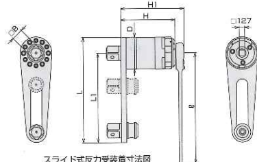
スライド式反力装着寸法図
